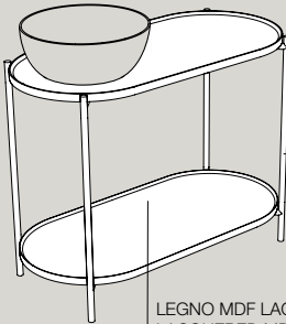
200S7607 struttura h 76 cm_frame h 76 cm 200R ripiano_shelf 100x48xh93 cm
