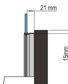
Detaliu A - vedere frontală
