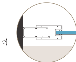
Fig. 1 Uși, Acces pe colț, Sfert de cerc
