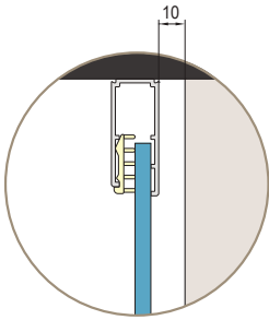
Fig. 2 Perete lateral
