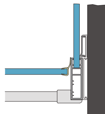
Detaliu A vedere de sus:
