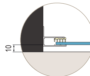
Fig. 2 Perete lateral
