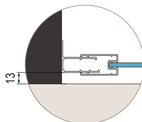
Fig. 1 Uși culisante D20S2, D20SE2 și D20SR.
