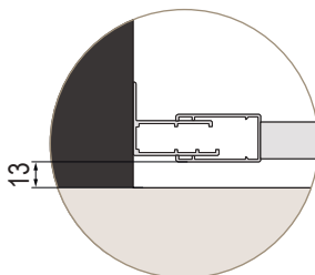
Fig. 1 Uși D20T1
