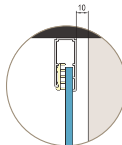
Fig. 2 Perete lateral
