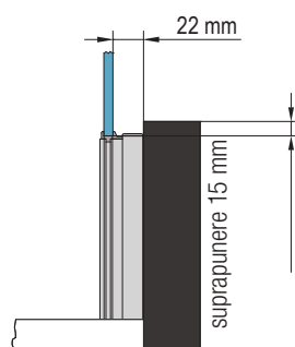
Detaliu A vedere frontală:
